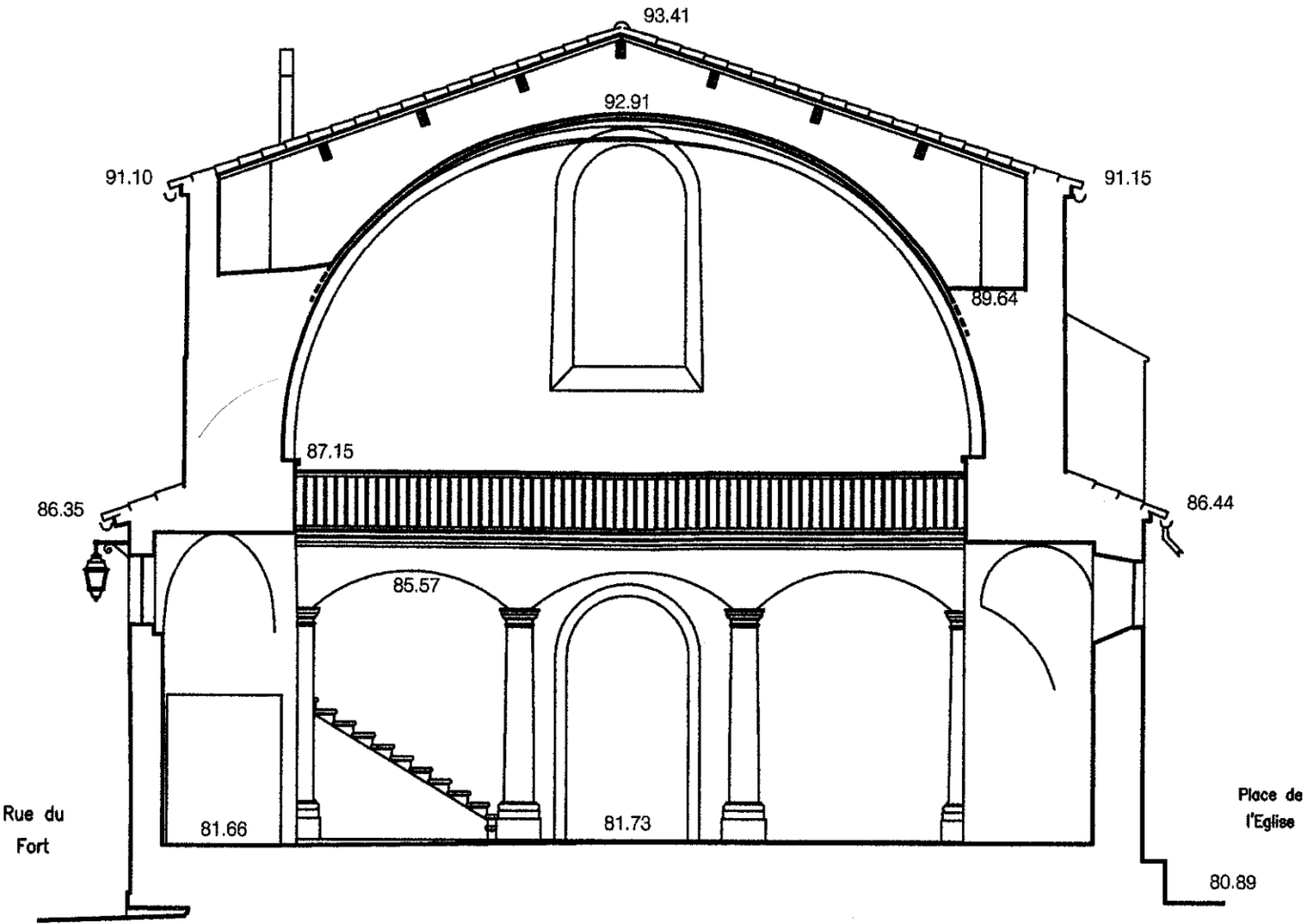
Coupe B-B
