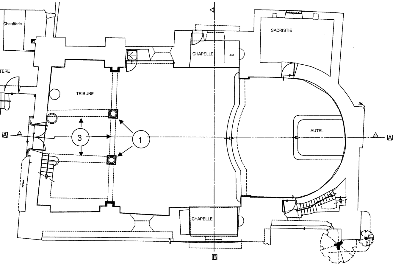
Plan du RDC
