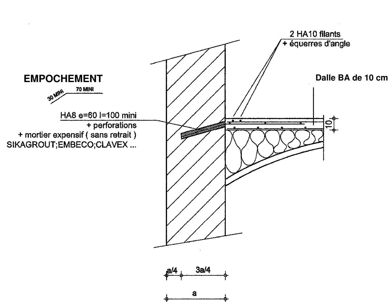
COUPE A - A
